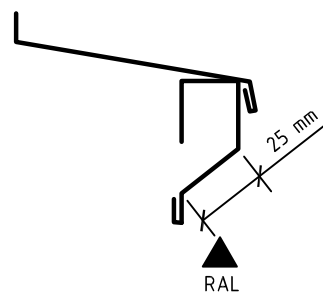
DETAIL OKAPNICE:
